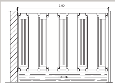
Façade avec cornadis sécurisé et porte pivotante à mi-hauteur (Prix à partir de CHF 1'542.80)
